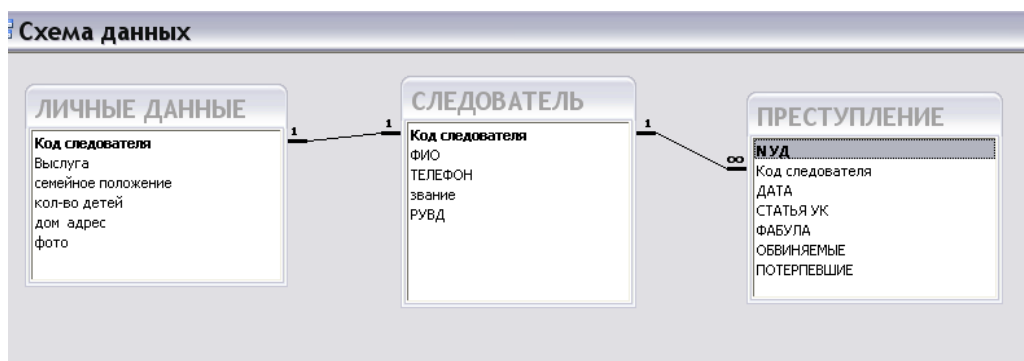
Рис. 5 Схема данных.
